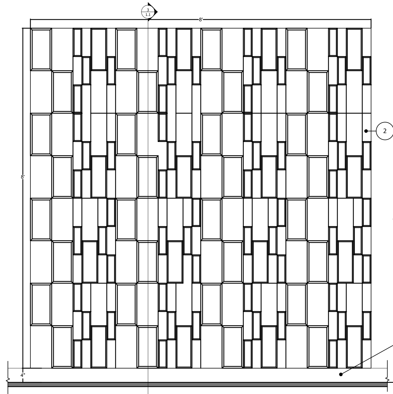
4 ELEVATION
