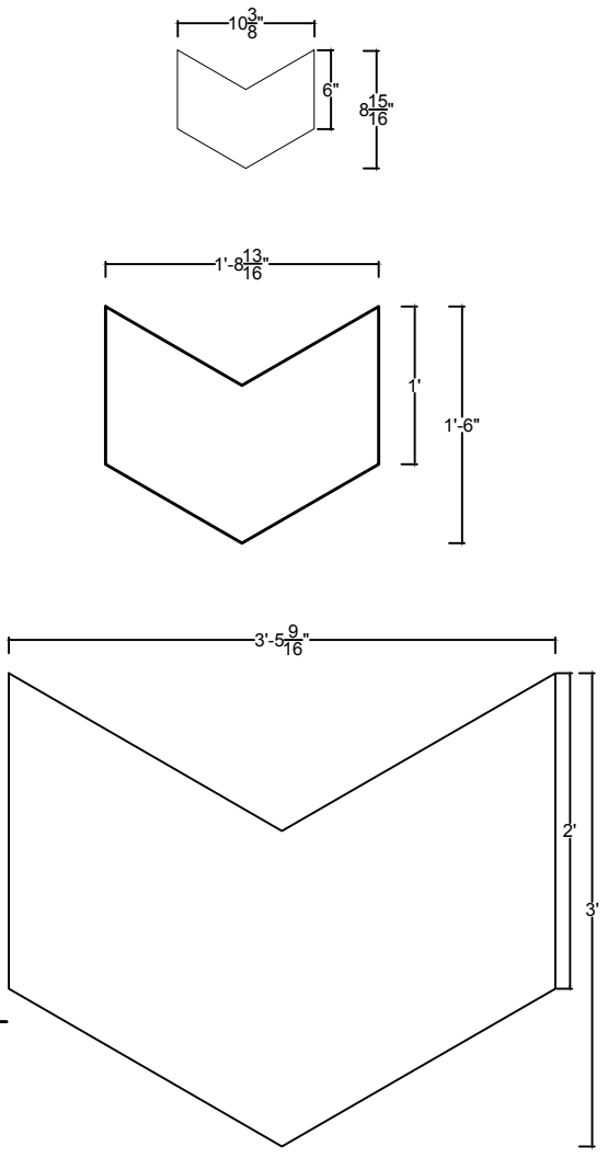
3 SECTION Scale: 3/4" = 1'-0"
