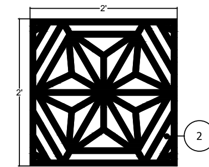
1 24" x 24" Scale: 3/4" = 1'-0"
