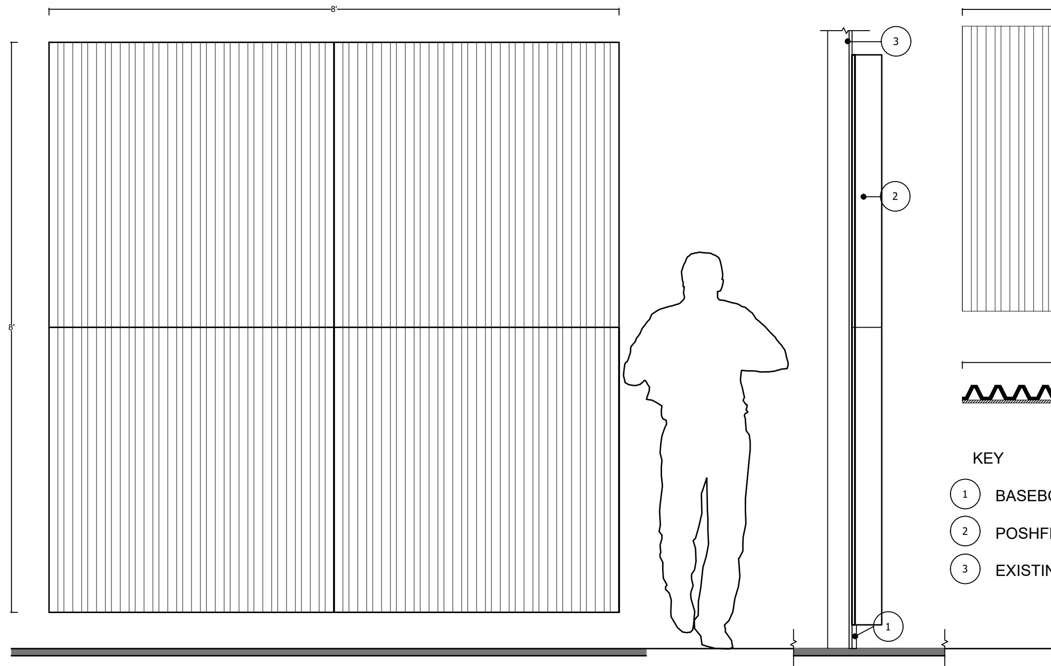
4 ELEVATION
