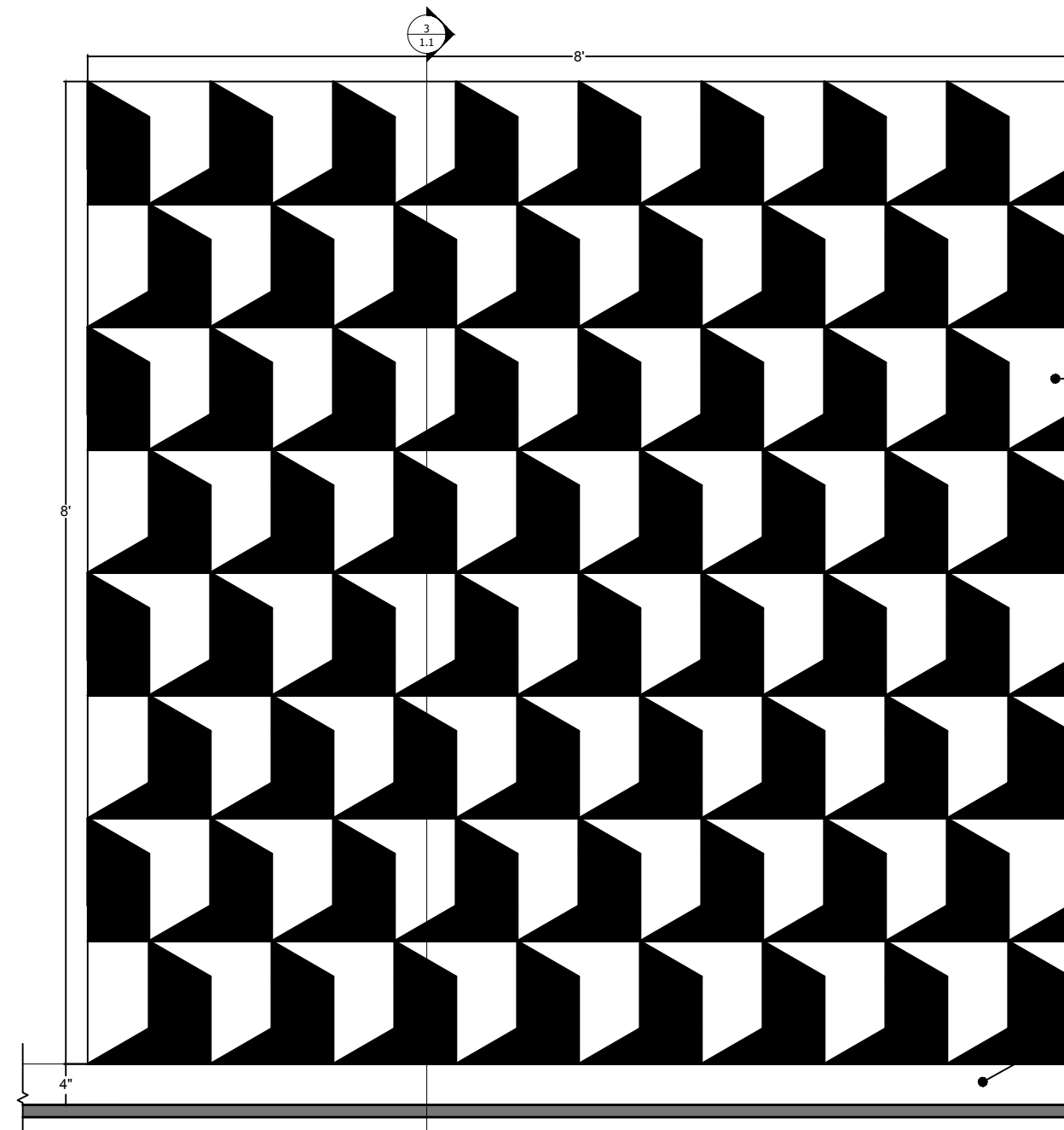
4 ELEVATION Scale: 3/4" = 1'-0"
