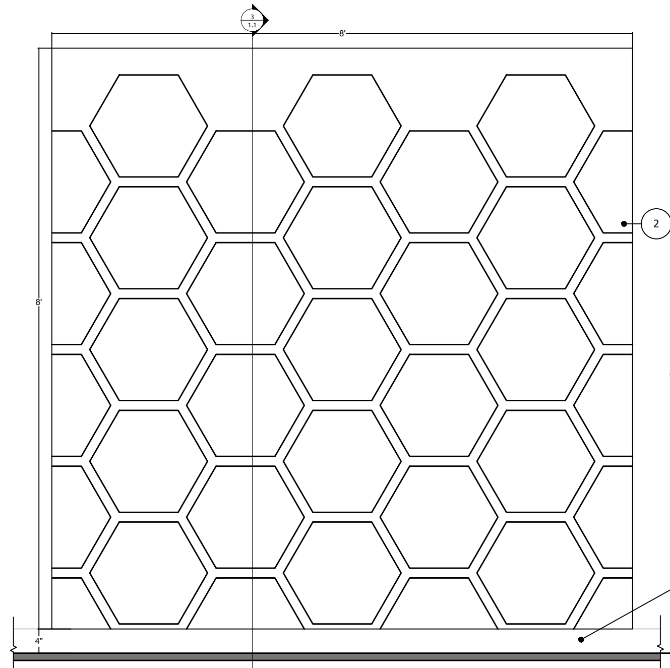
4 ELEVATION Scale: 3/4" = 1'-0"
