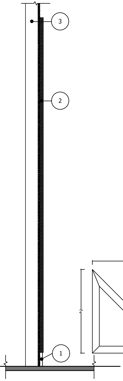
3 SECTION Scale: 3/4" = 1'-0"
