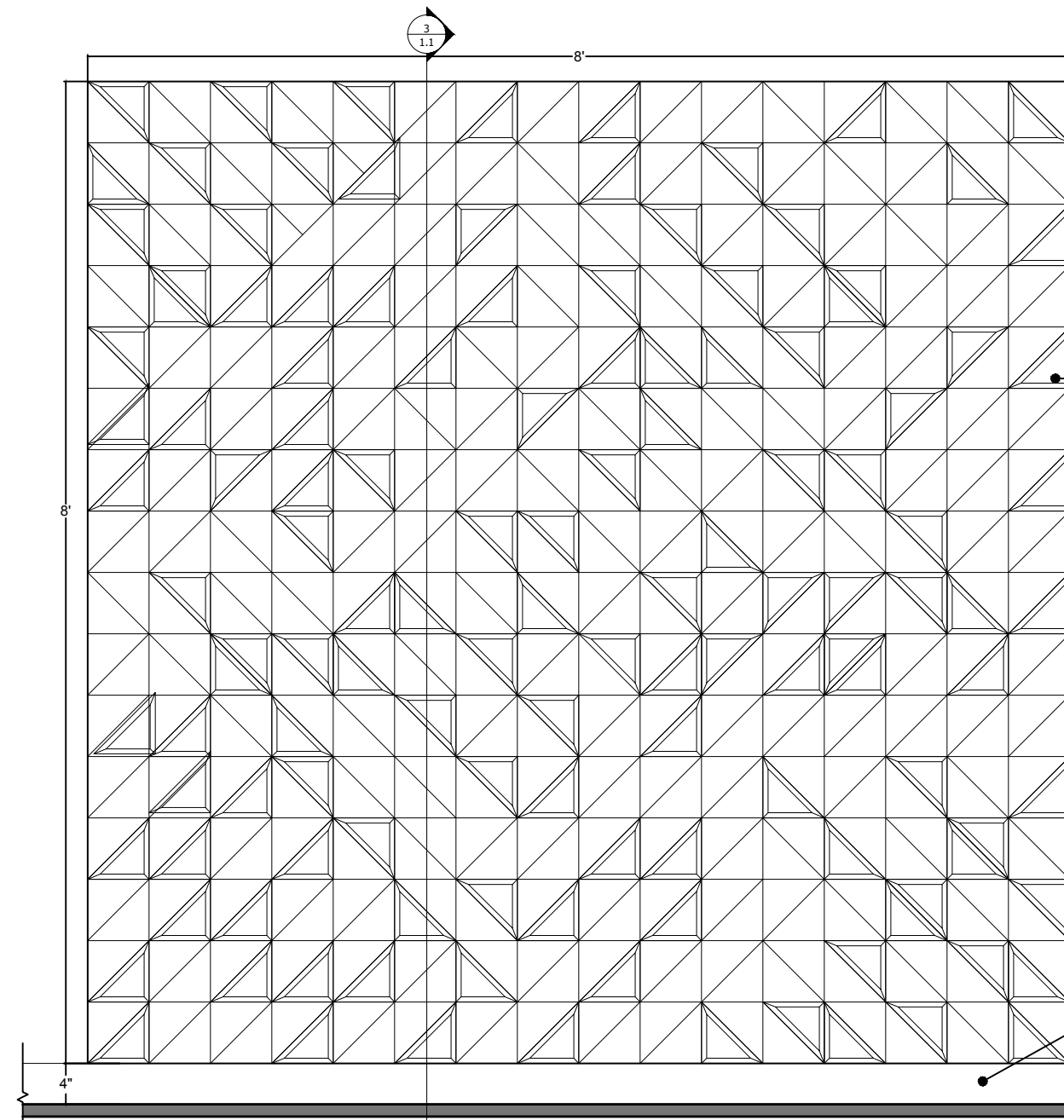
4 ELEVATION Scale: 3/4" = 1'-0"
