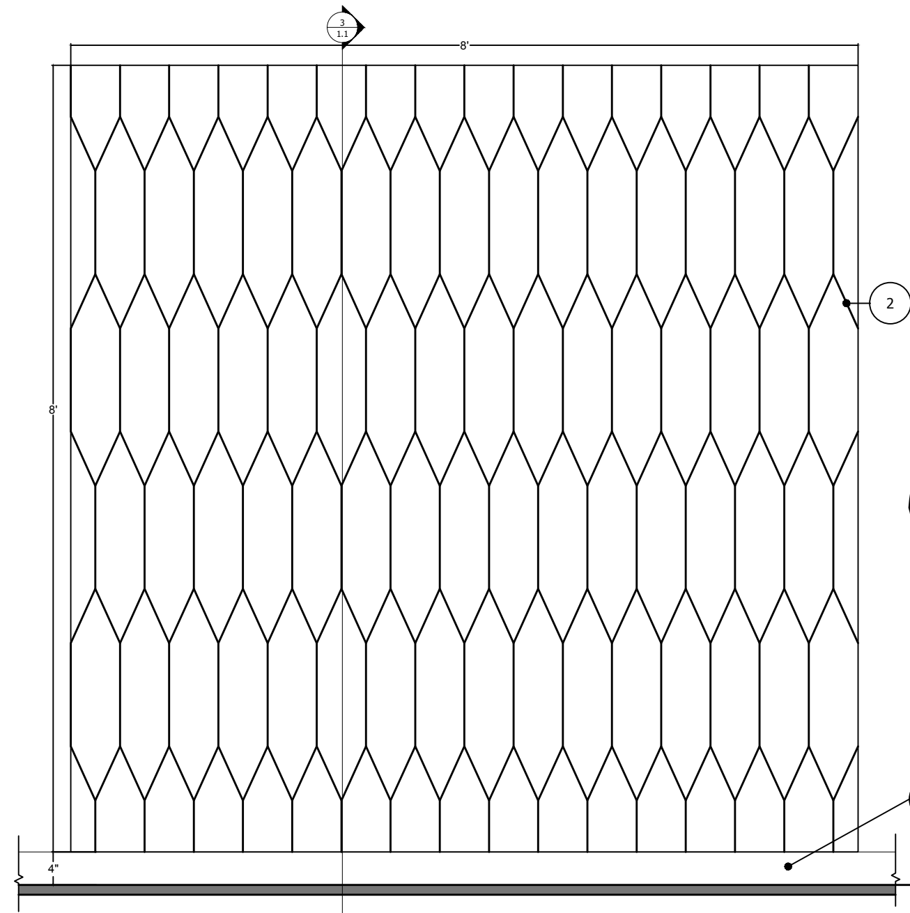
4 ELEVATION Scale: 3/4" = 1'-0"
