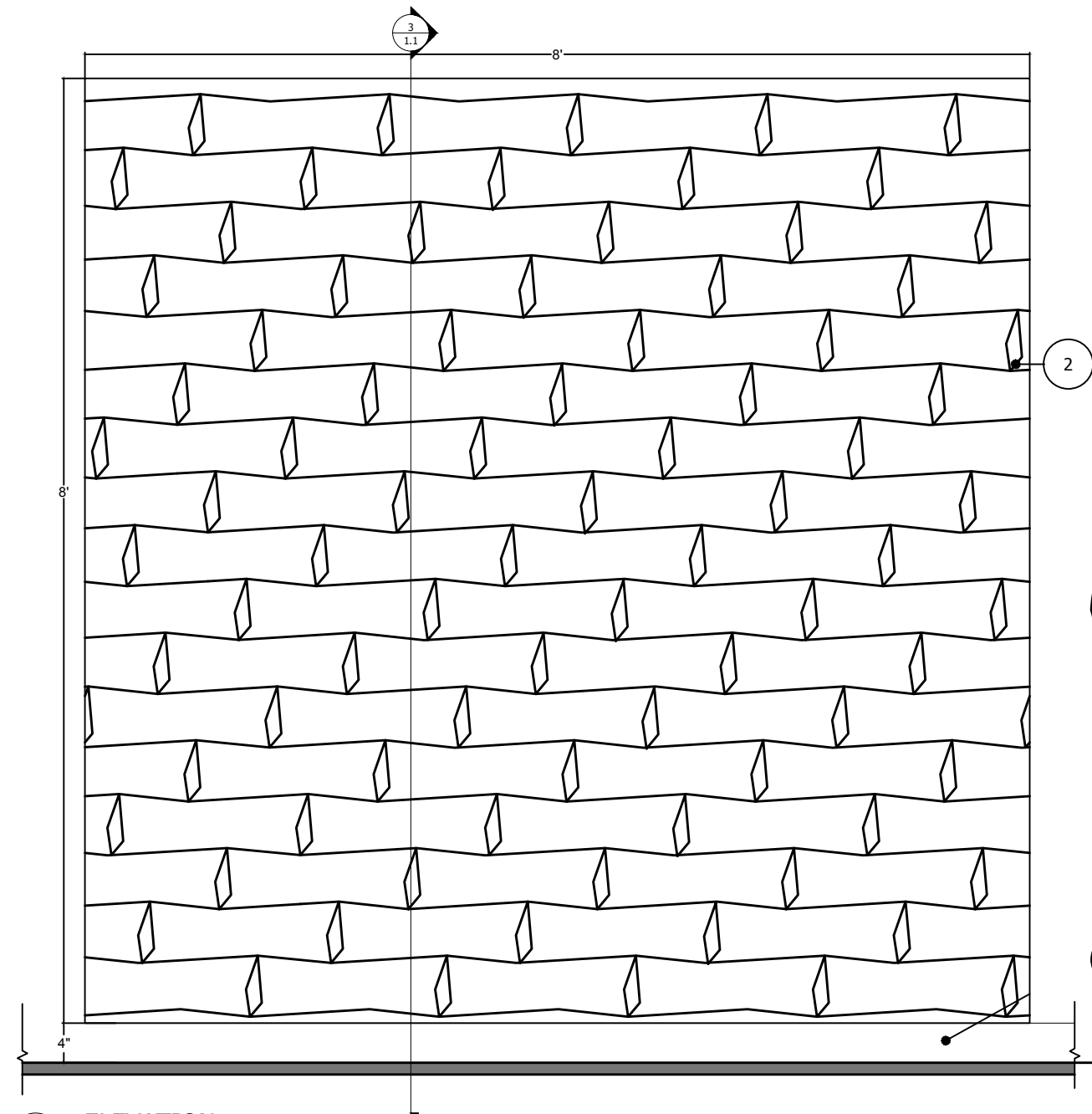
4 ELEVATION Scale: 3/4" = 1'-0"
