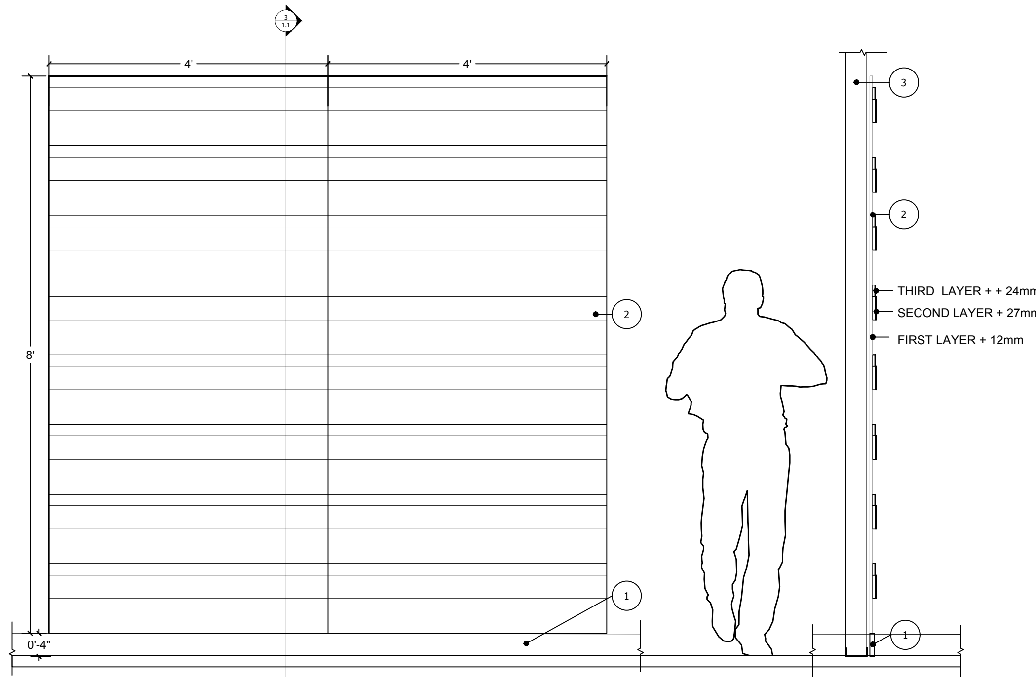
4 SLAT DEPTH ELEVATION
