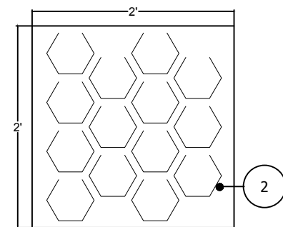
1 24" x 24" Scale: 3/4" = 1'-0"
