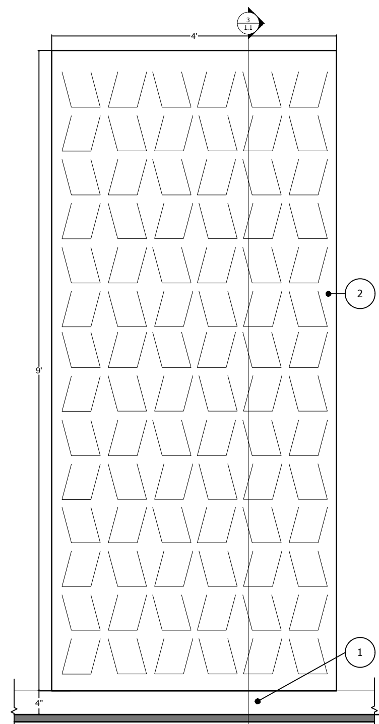
4 ELEVATION Scale: 3/4" = 1'-0"
