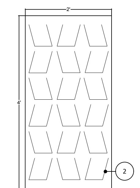
2 48" x 24" Scale: 3/4" = 1'-0"
