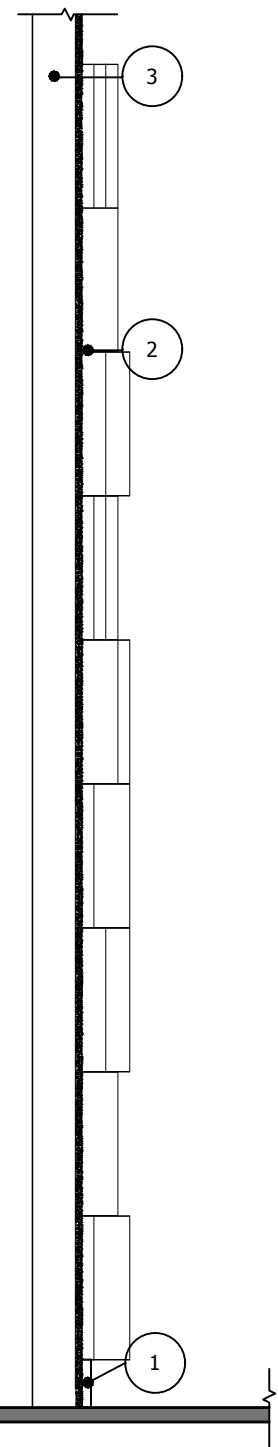
3 SECTION Scale: 3/4" = 1'-0"
