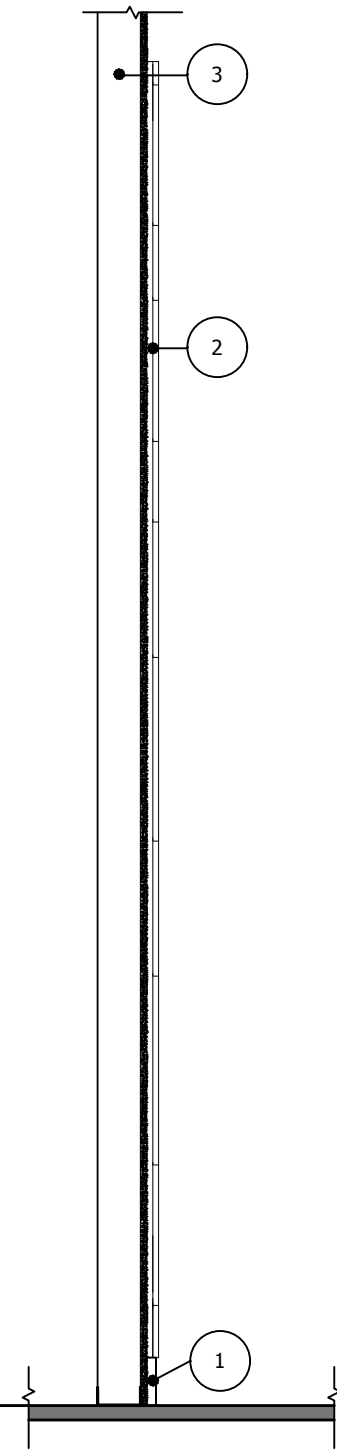
3 SECTION Scale: 3/4" = 1'-0"
