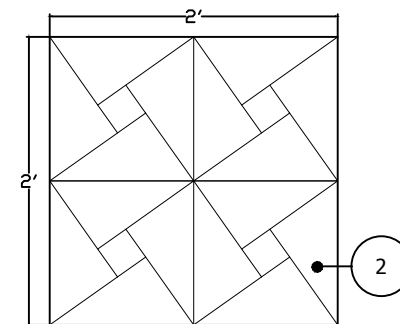
1 24" x 24" Scale: 3/4" = 1'-0"
