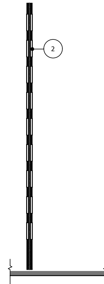
3 SECTION Scale: 3/4" = 1'-0"
