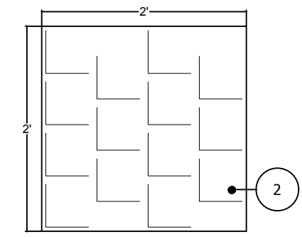
1 24" x 24" Scale: 3/4" = 1'-0"
